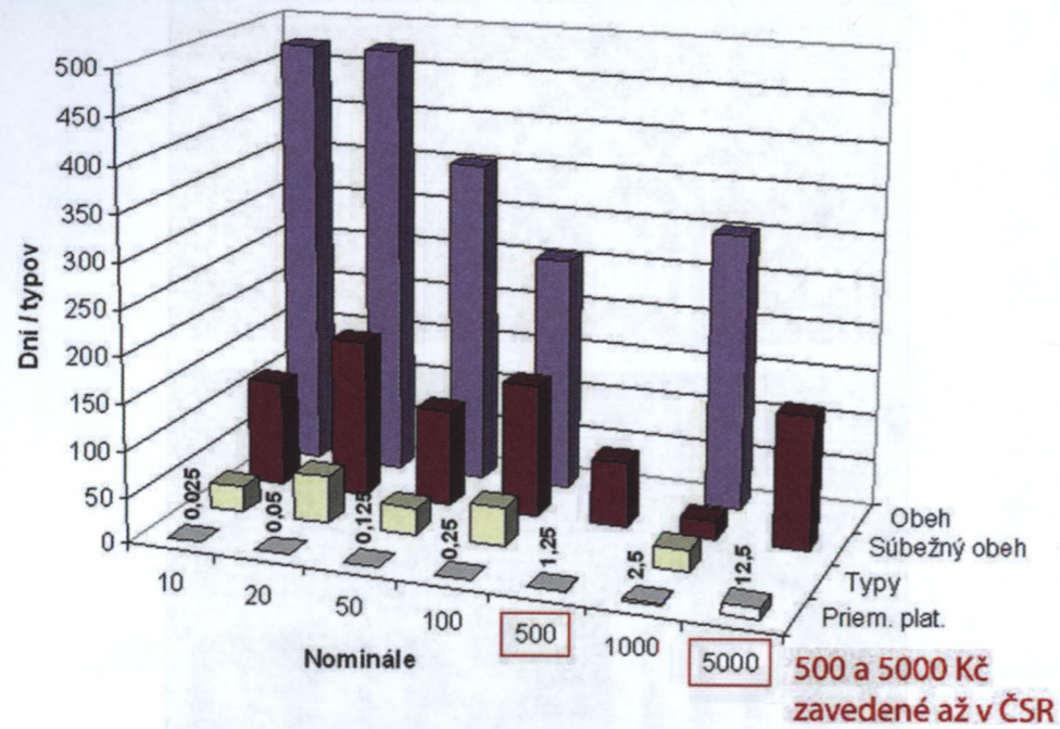
Závislosť počtu typov falšovaných kolkov na nominále štátovky, dĺžke je obehu a dĺžke súbežného obehu s bankovkou rovnakého alebo blízkeho nominále.
